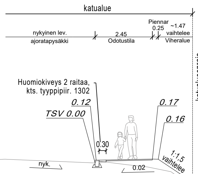
Tyyppipoikkileikkaus A - A
