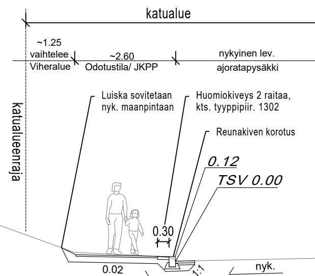
Tyypipoikkileikkaus A - A
