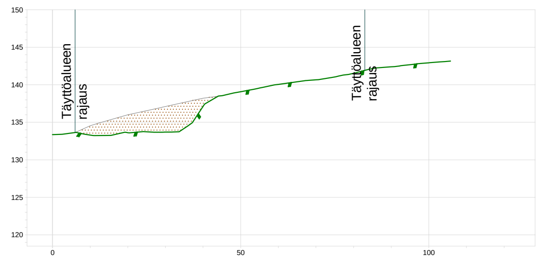
Pituusleikkaus
