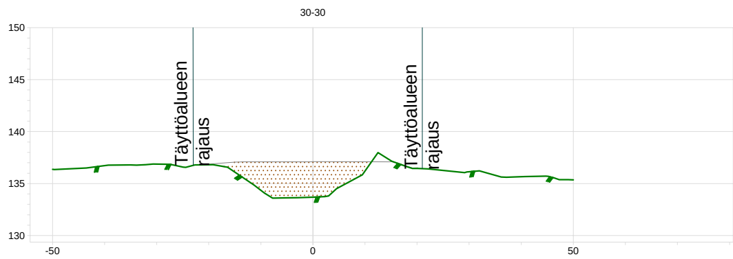
Poikkileikkaukset
