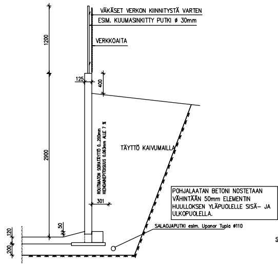
LEIKKAUS 1-1
