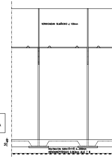
LEIKKAUS 2-2
