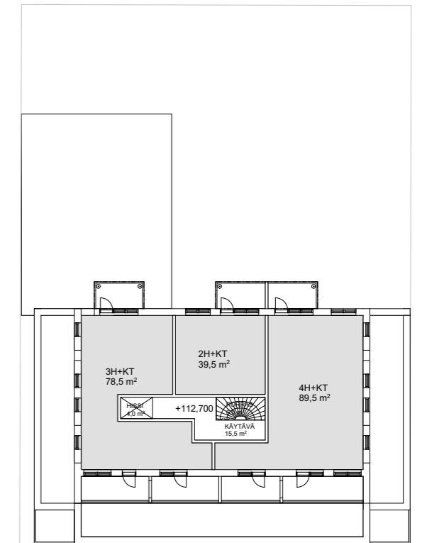
Suokatu 23, 7. kerros 1:400
