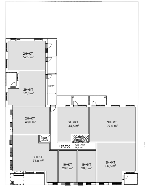
Suokatu 23, 2. kerros 1:400
