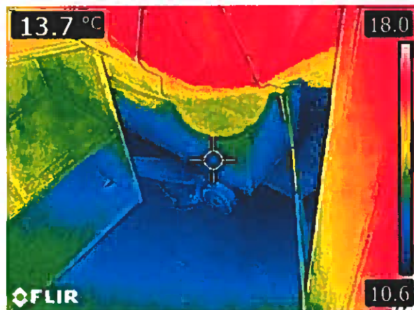
Kuva 7. Lepotilan 116 kaapin ja ulkoseinän liittymäpinnat ovat viileät (ilma- ja lämpövuotoja).
