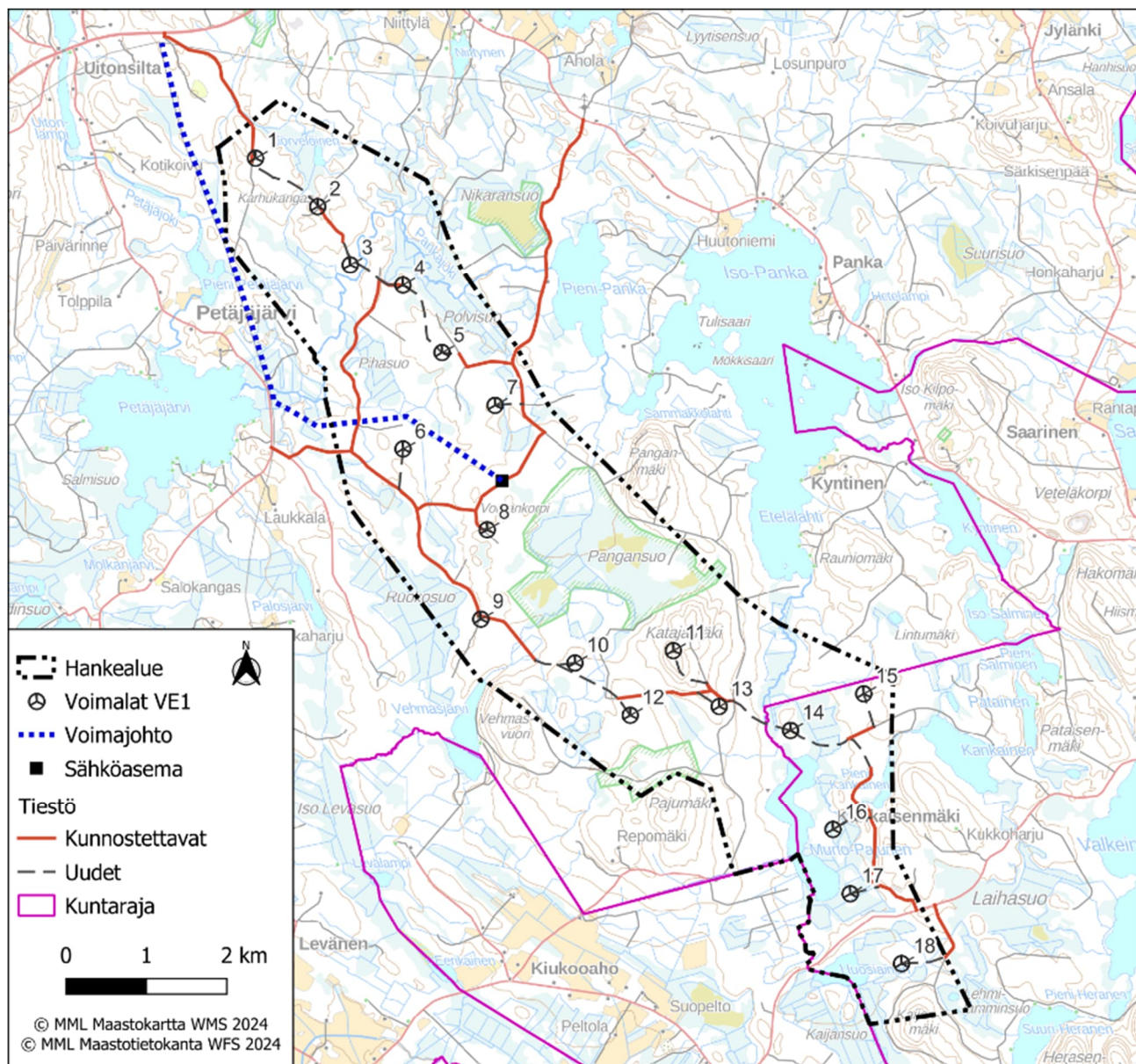
Kuva 2. Vornankorven tuulivoimapauston voimalasijoittelu hankevaihtoehdossa VE1.
