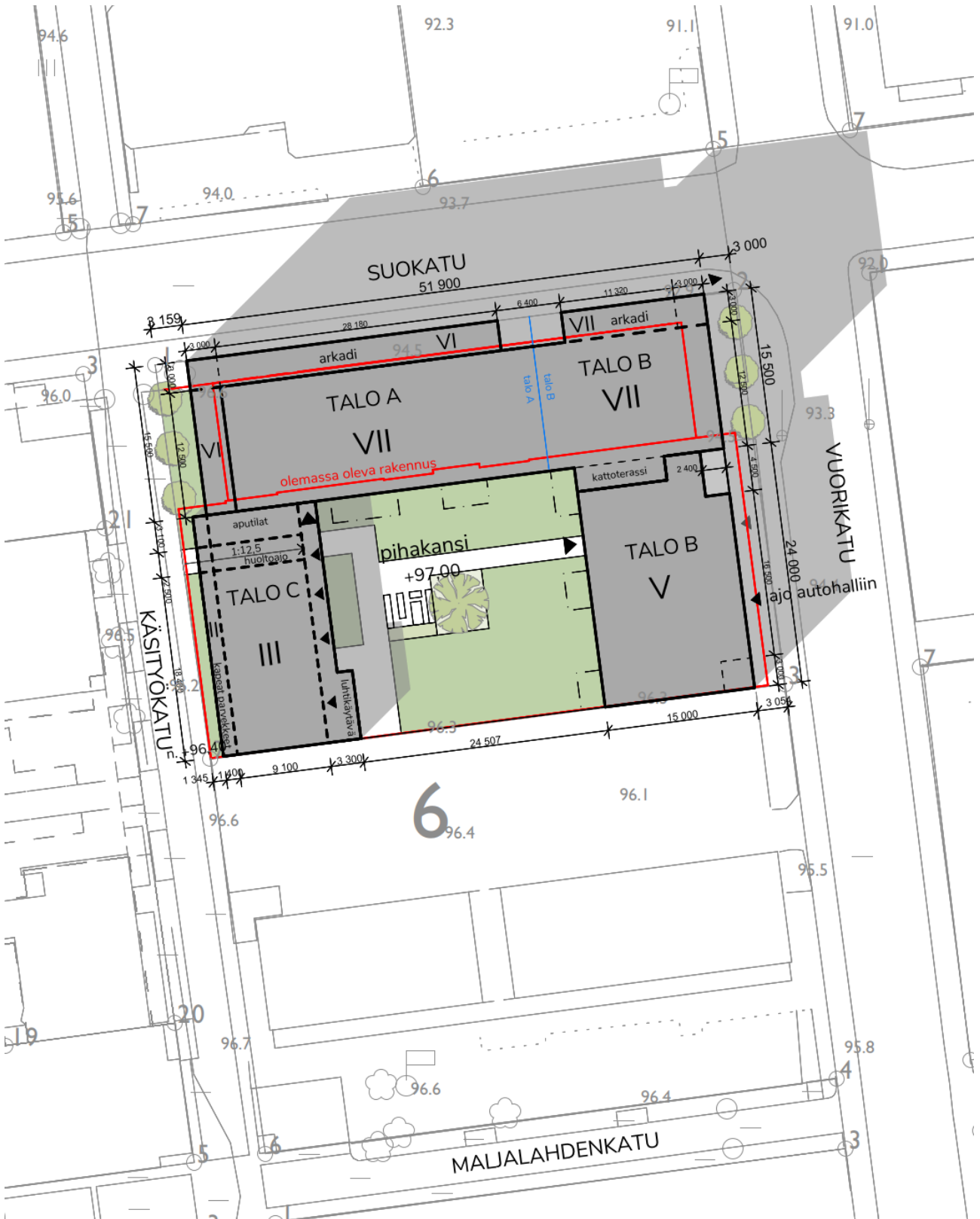
Kuva 46. Asemapiirustus. Punaisella viivalla nykyisen rakennuksen ulkorajat.
