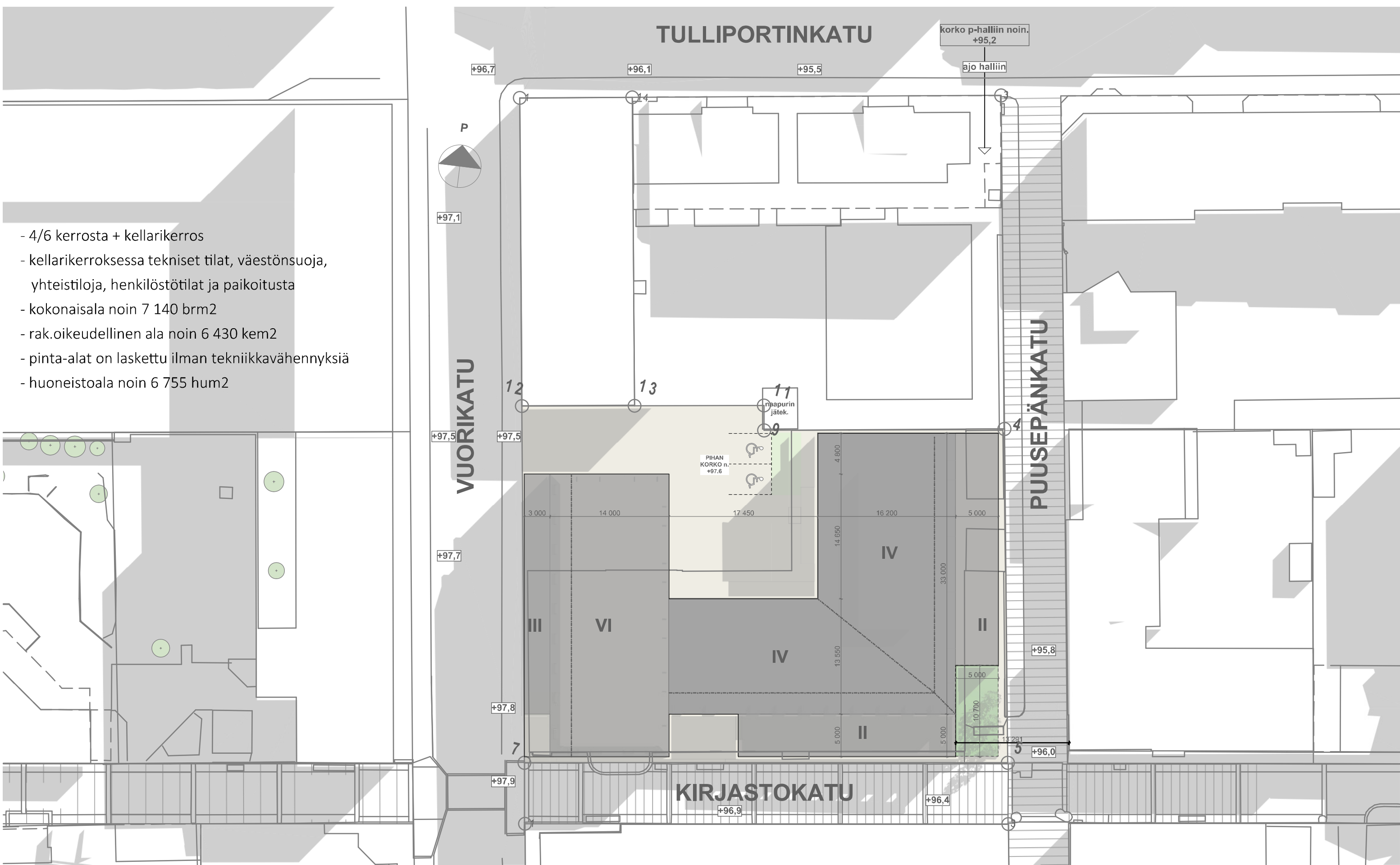
VE3 ASEMAPIIRROS 1:500
