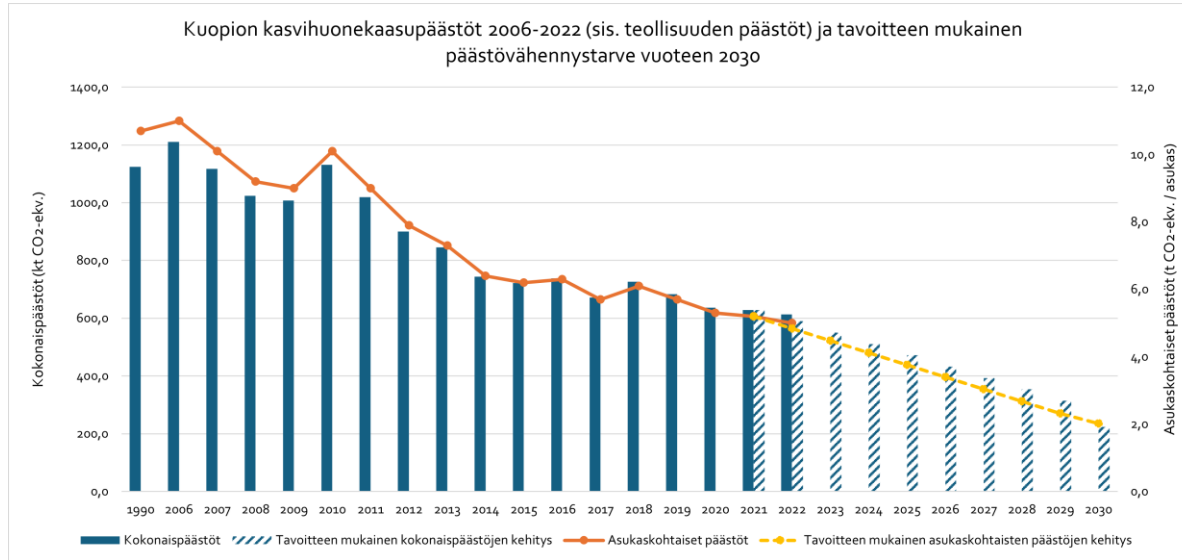
Kuva 6: Kuopion kasvihuonekaasupäästöt vuosilta 2006-2022 sisältäen teollisuuden päästöt (lähde: Kuopion CO 2 -raportti 2024, Sitowise) sekä päästövähennystavoitteen mukainen päästövähennystarve vuoteen 2030 saakka.
