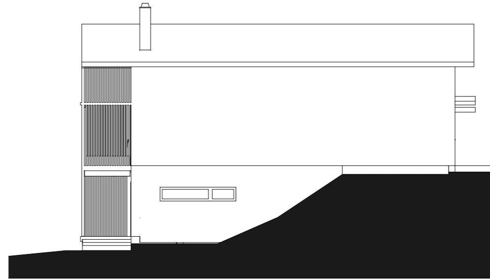
Julkisivu etelään
