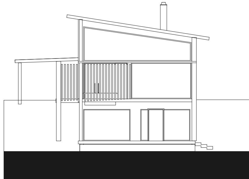
Julkisivu länteen
