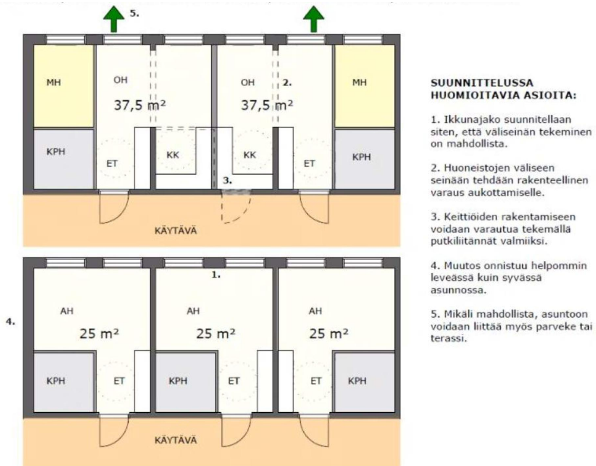
Kuva 9 ARA:lla on menossa hanke, jossa tutkitaan tehostetun palveluasumisrakennusten muuntojoustavuutta esim. palvelutaloiksi. Muuntojoustoon voidaan vaikuttaa rakennerratkaisuin ja tekniikan nousuvarauksin
