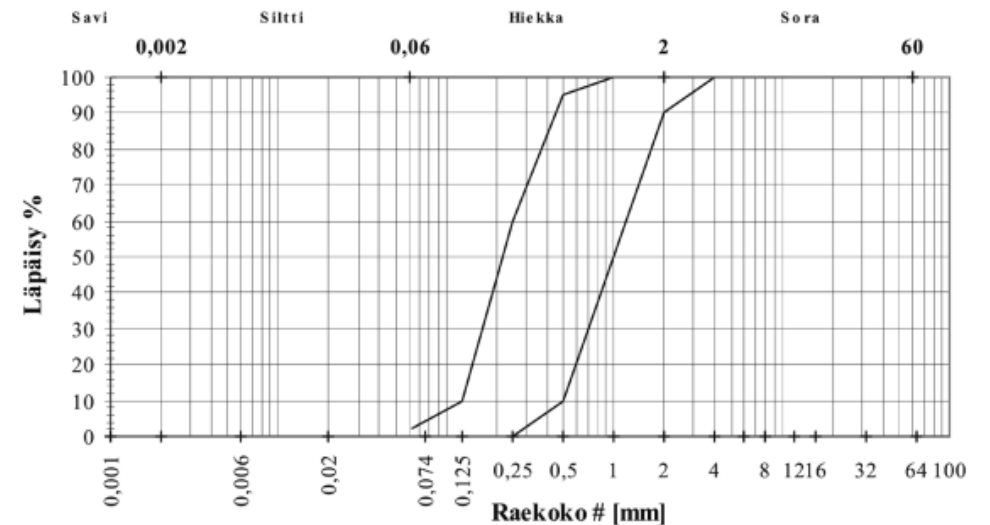
Kuva 7. Beach volley -kentän hiekan rakeisuuden ohjealue.
