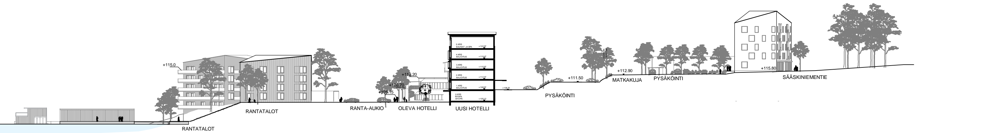
Alueleikkaus rannasta Säaskiniementielle hotellin jaajennukseen kohdalta
