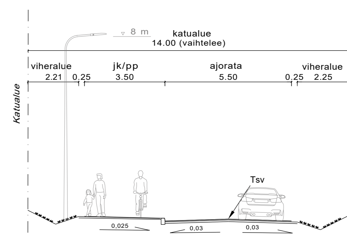
Tyyppipoikkileikkaus 2a-2a
