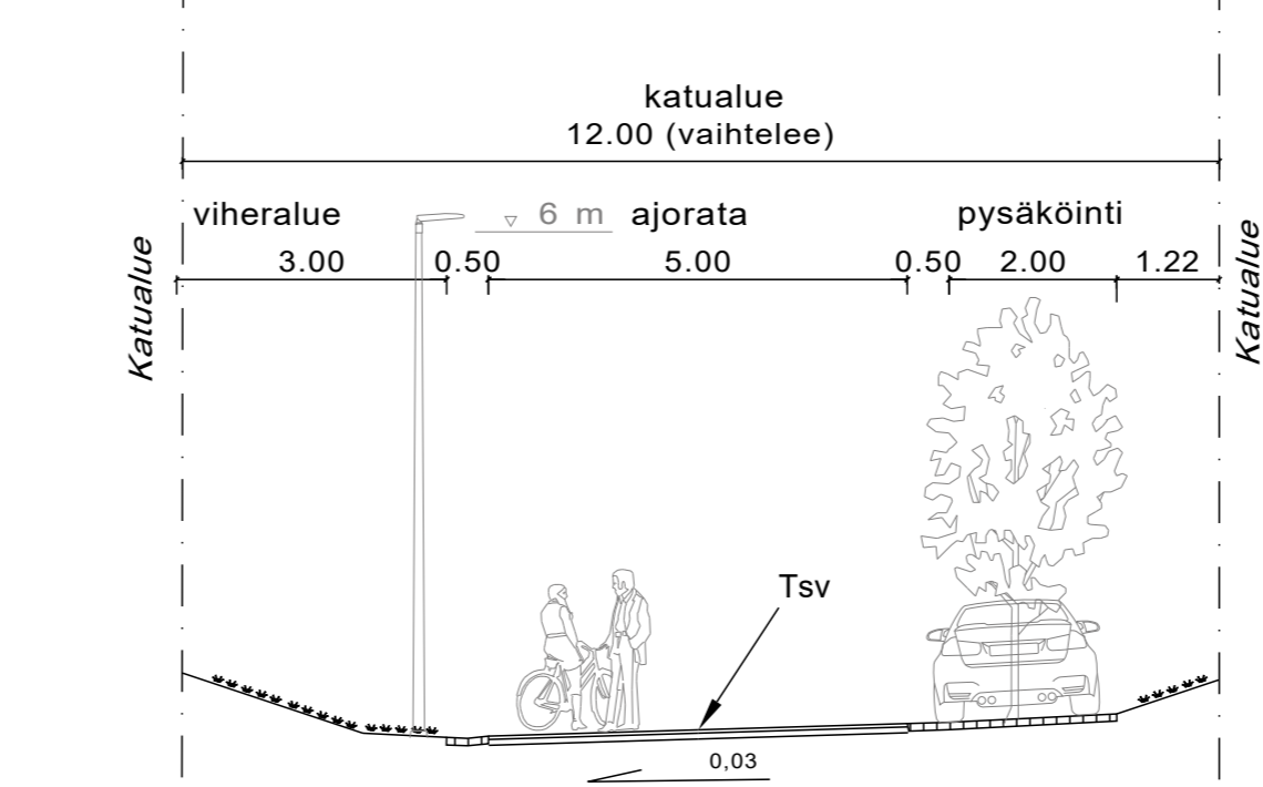
Tyyppipoikkileikkaus 2a-2a
