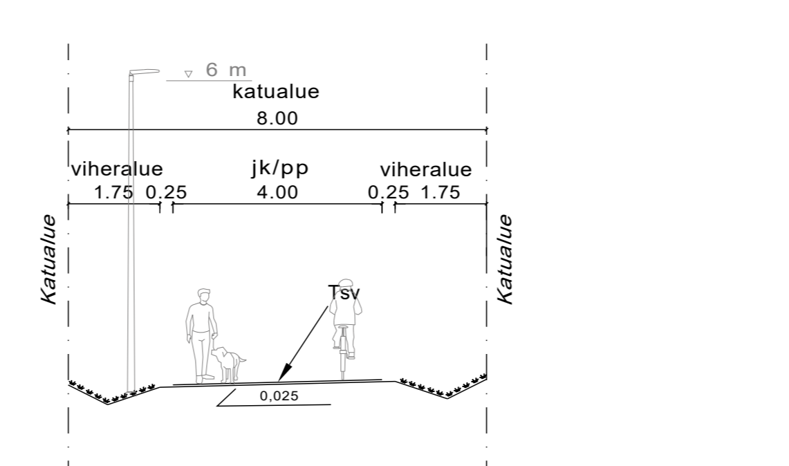
Tyyppipoikkileikkaus 3-3
