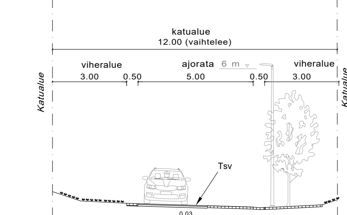
Tyyppipoikkileikkaus 2b-2b
