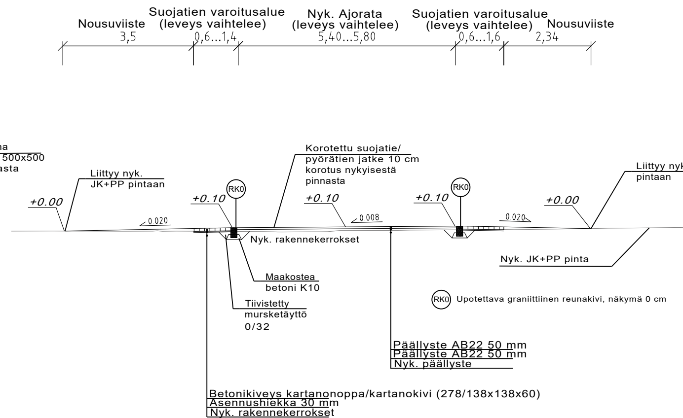
Tyypipoikkileikkaus Leikkaus B-B
