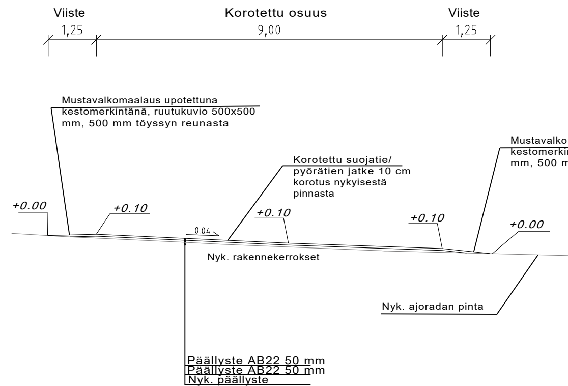
Tyypipoikkileikkaus Leikkaus A-A
